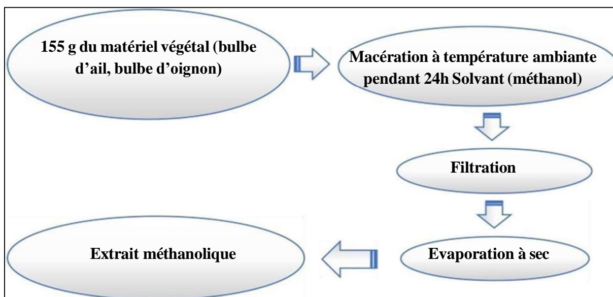
Figure 02 : Protocole d'extraction par macération d'ail et d'oignon.
