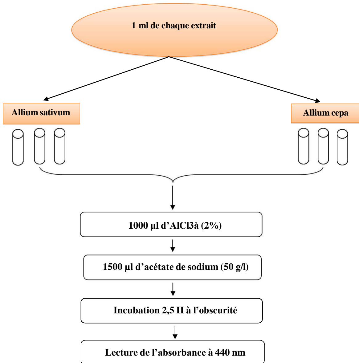
Figure 06 : Protocole de dosage des flavonols totaux
