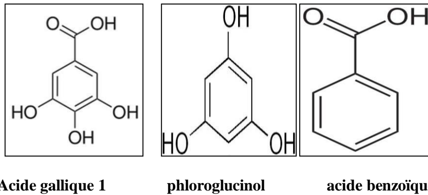
Figure 04 : Quelques phénols et acides phénoliques
