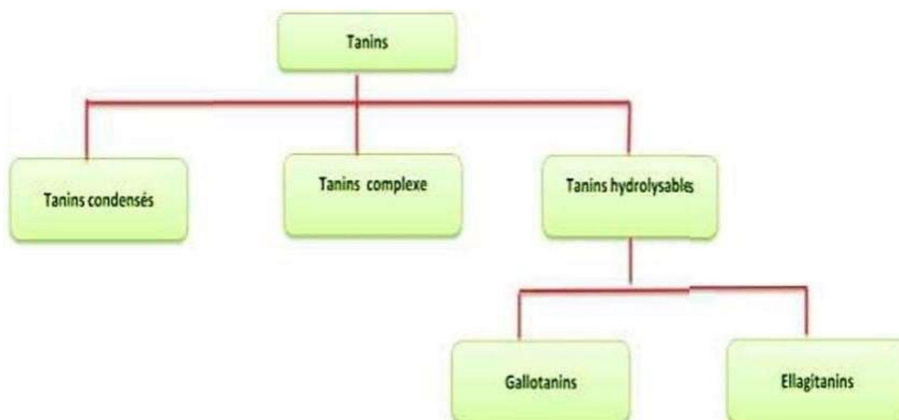
Figure 06 : Classification des tanins (Vermerris et Nicholson, 2006).
