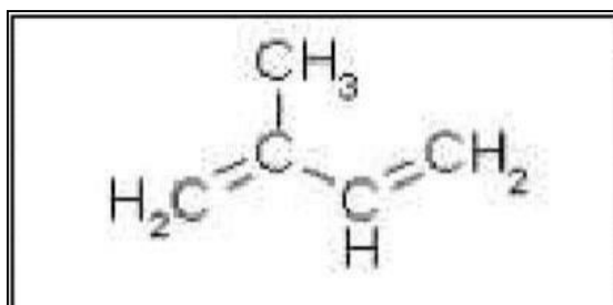
Figure 12 : Molécule d'isoprène (Malecky, 2008).
