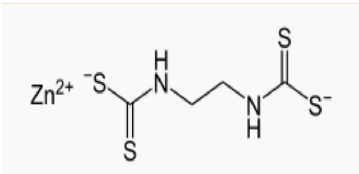
Figure 11 : Structure chimique de Zinèbe.
