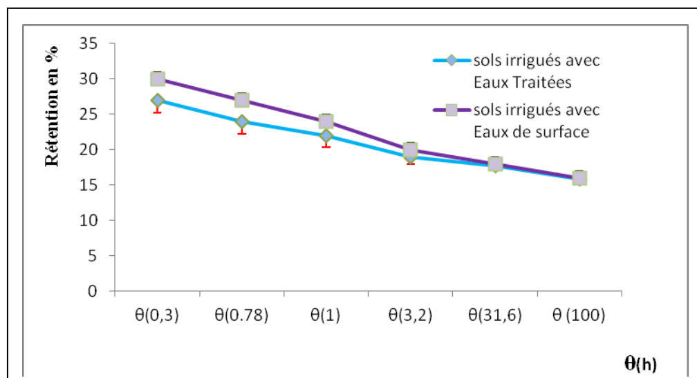
Fig.6. Courbes de rétention d'eau pour les sols irrigués avec les deux types d'eau (ET : sols irrigué à l'eau traitée, ES : sols irrigué à l'eau de surface)
