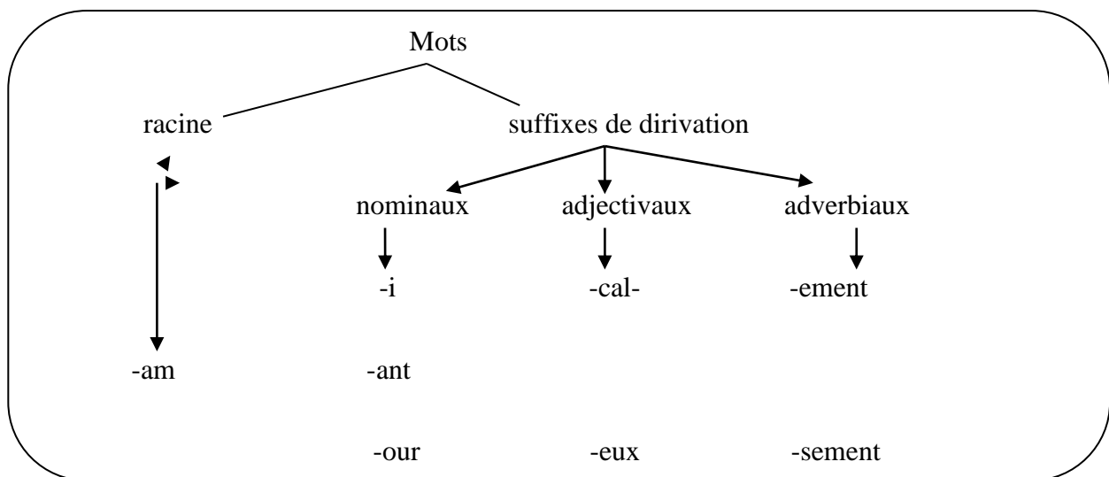
Figure 1: mots dérivés de la racine am- [38]
