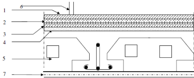
Figure II-8 : Composants d'un plancher étage courant corps creux.
