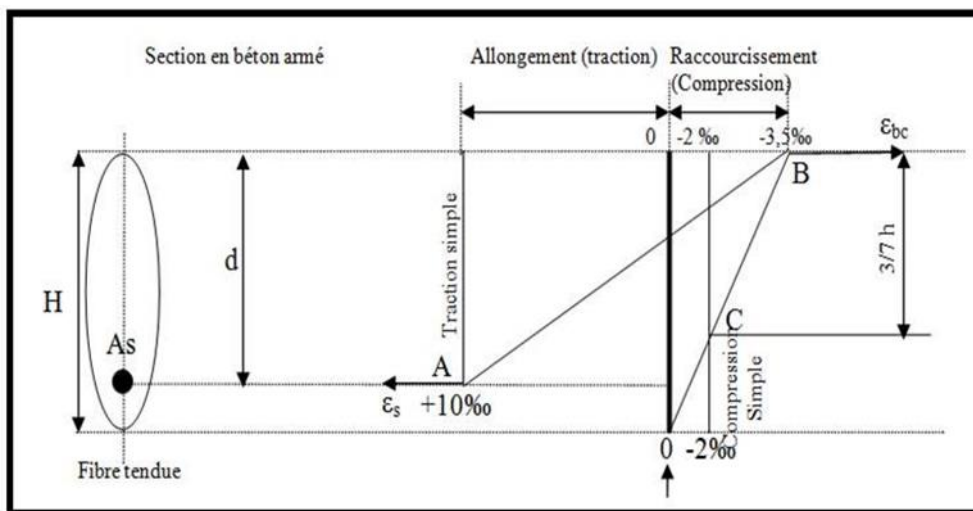
Figure I-6 : Diagrammes des déformations limitées de la section.
