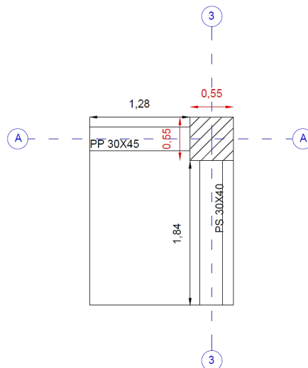
FigureII-14 : Poteau d'angle A1.
