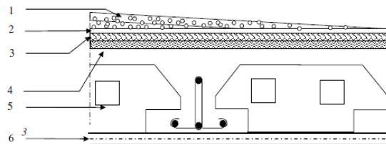
Figure II-7 : Composants d'un plancher terrasse accessible en corps creux.
