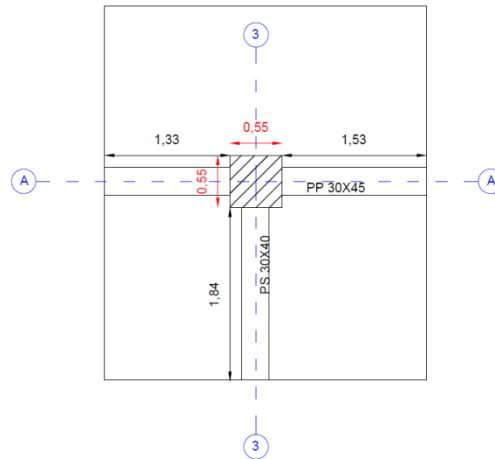
FigureII-13 : Poteau de rive A3.
