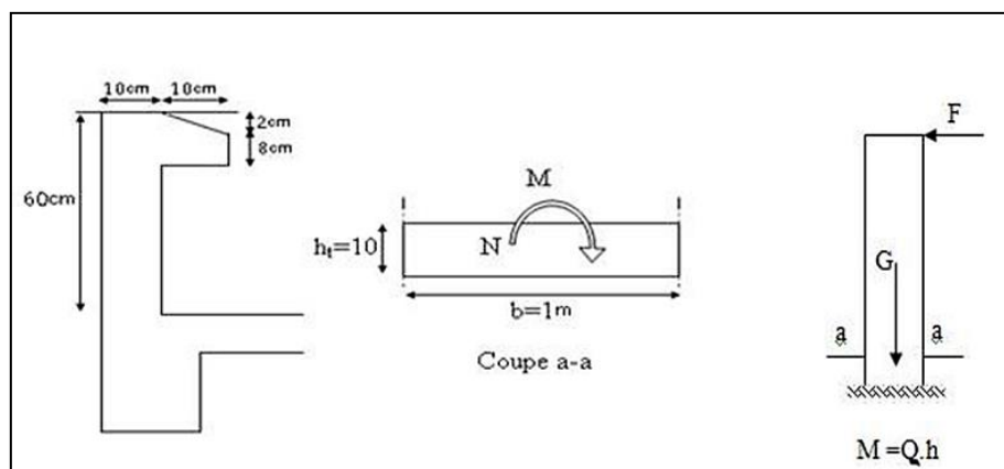
Figure III-1 : Schéma l'acrotère.
