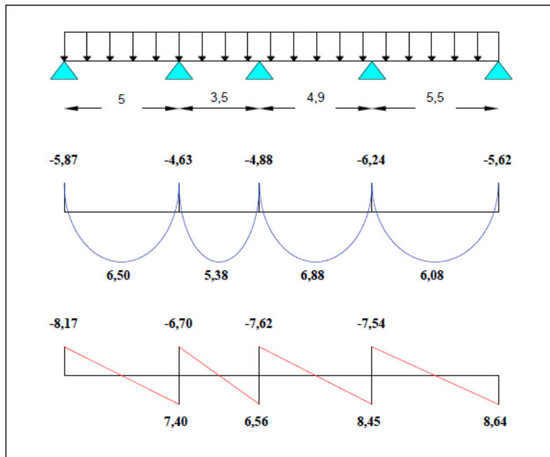
Figure III-7 : Diagrammes des moments entravés et efforts tranchants à l'ELU.
