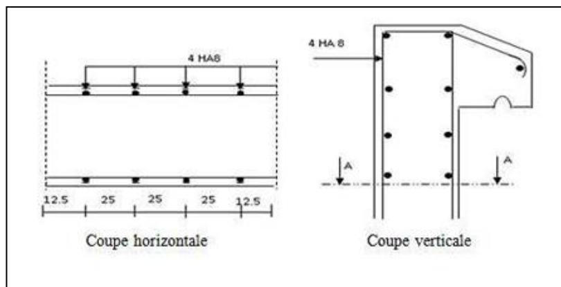
Figure III-2:Schéma de ferrailage
