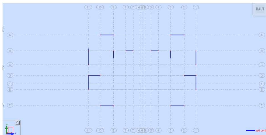
Figure V-9 : Disposition des voiles dans la zone sismique 03.
