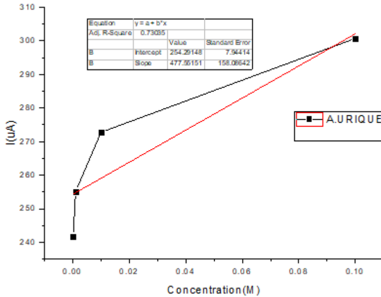
Figure II.12: Courbe d'étalonnage relatif à la détection d'acide urique par NIP
