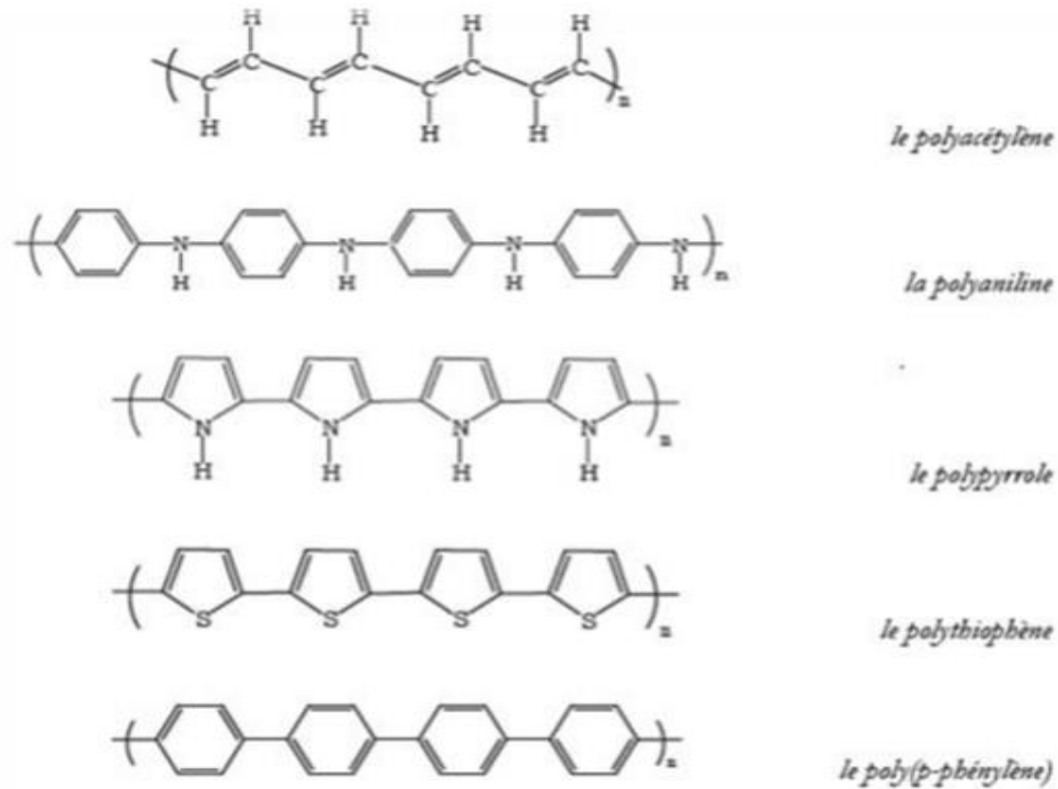
Figure 0.14: Exemple de quelques polymères conducteurs
