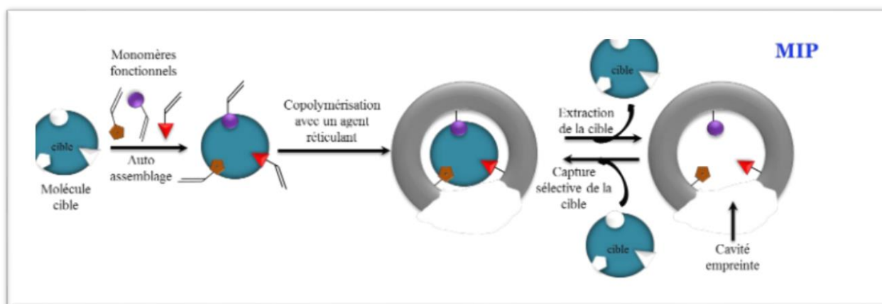
Figure 0.13: Principe des polymères à empreintes moléculaires
