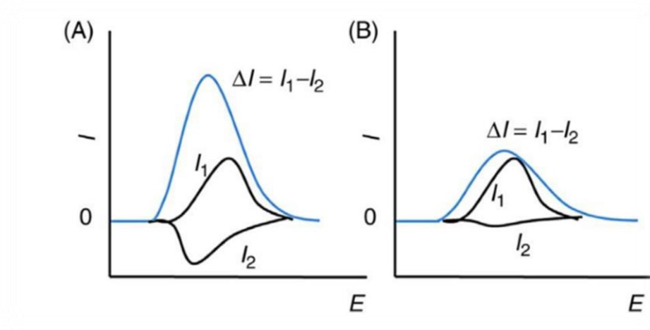
Figure 0.11: Schématisation d'un Voltammogramme à onde carrée, où : (A) pour un processus redox d'un système réversible et (B) représente celui d'un système irréversible [39]
