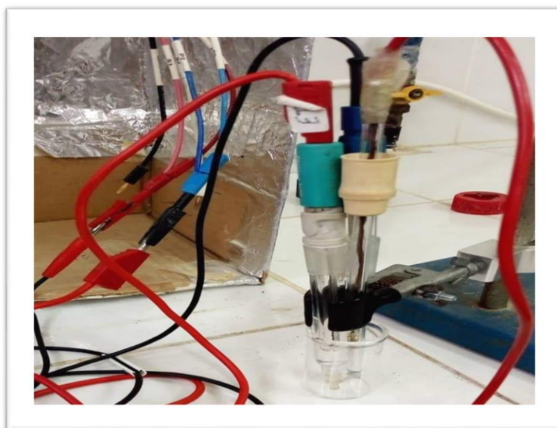
Figure 0.18 : cellule électrochimique a trois électrodes Les Un système à trois électrodes
