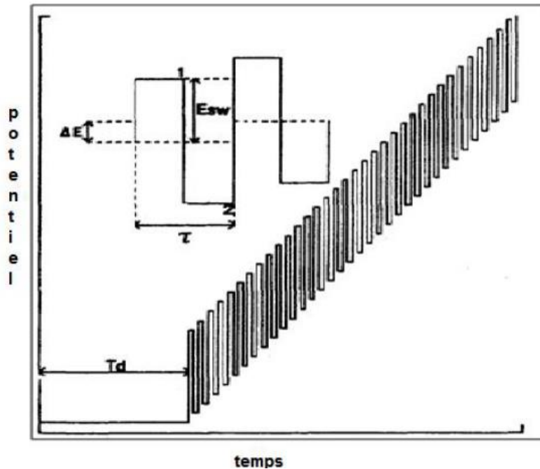
Figure 0.10 : Variation de potentiel en fonction du temps d'un Voltammogramme à onde carré [36]
