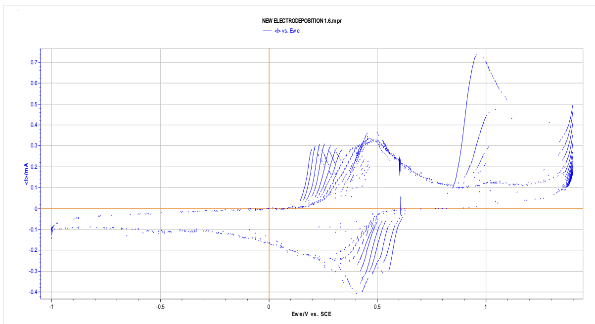
Figure 0.22: Voltammogramme cycliques successifs d'électrodéposition obtenue avec une électrode de CARBONE VITREUX/NET/PAN dans une solution de \text{H}_2\text{SO}_4 (0.1M).
