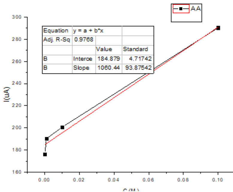
Figure III.15 : Courbe d'étalonnage relatif à la détection d'acide urique par MIP
