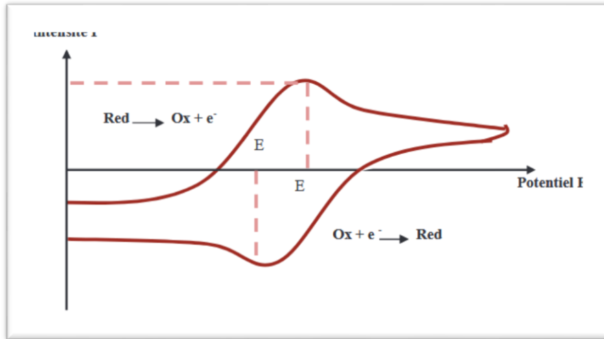
Figure 0.9: Exemple d'un voltampérogramme cyclique pour un système lent
