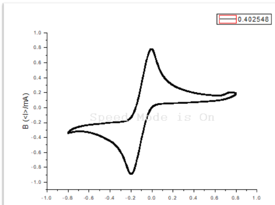
Figure 0.21: Voltammogramme de l'électrode de carbone vitreux), en milieu contenant 5mM de K_3[Fe(CN)_6]/K_4[Fe(CN)_6] ; v = 50 mV/s
