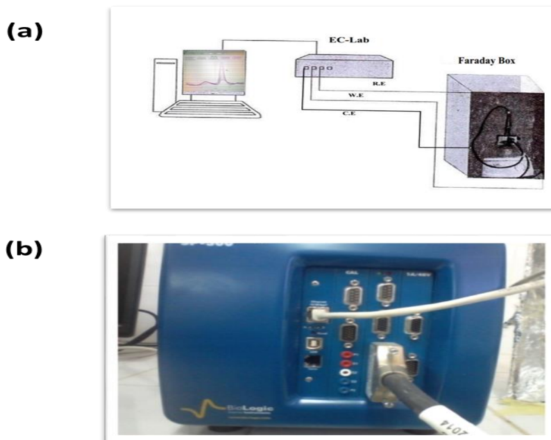
Figure 0.19 : (a) Schéma de la diapositive expérimental pour les mesures électrochimiques (EC-Lab), (b) photographie de l'appareil
