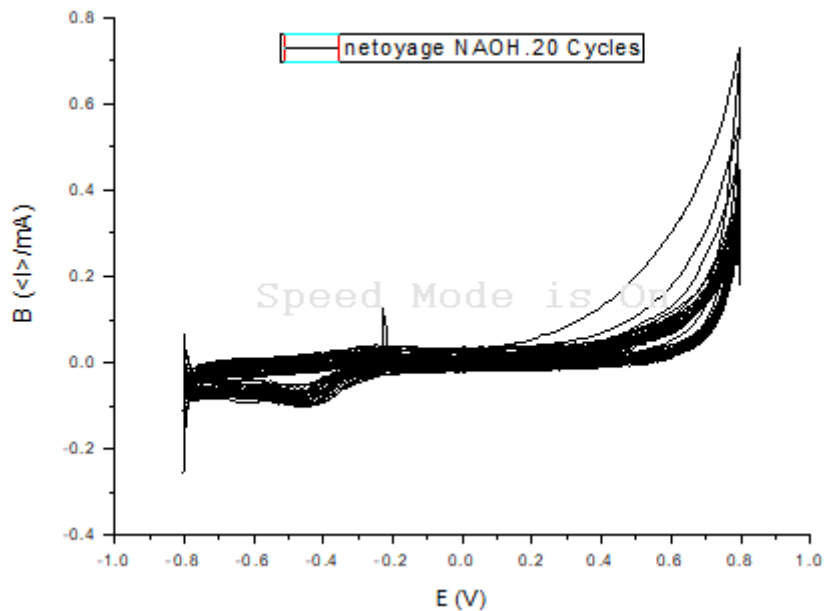
Figure 0.20 : Voltammogramme relatifs à l'activation par 20 cycles d'une électrode de carbone vitreux dans une solution de NaOH (0.5M) a V=50 mV/s
