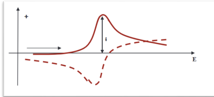
Figure 0.7: Voltammogramme cyclique d'un couple redox (système réversible)
