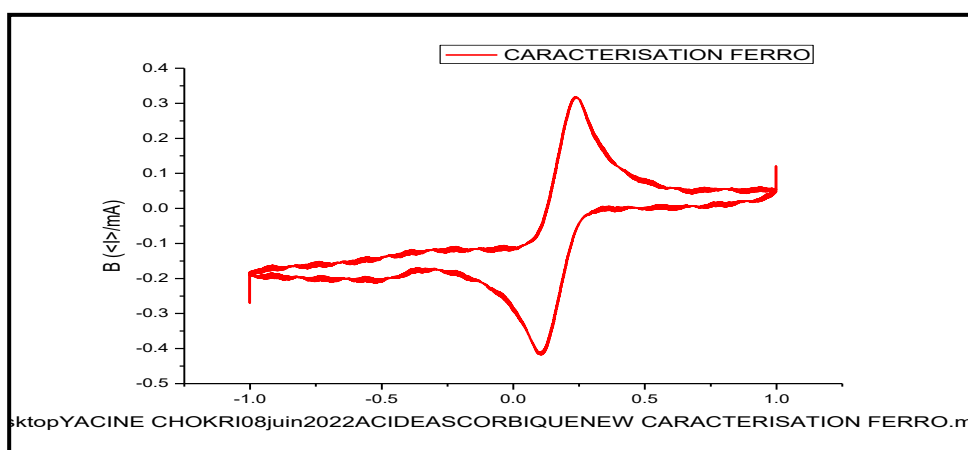
Figure.III.13 : Caractérisation par SQW du capteur vis-à-vis d'acide urique
