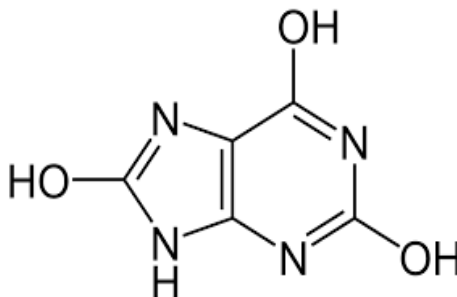
Figure 0.16 : structure de l'acide urique
