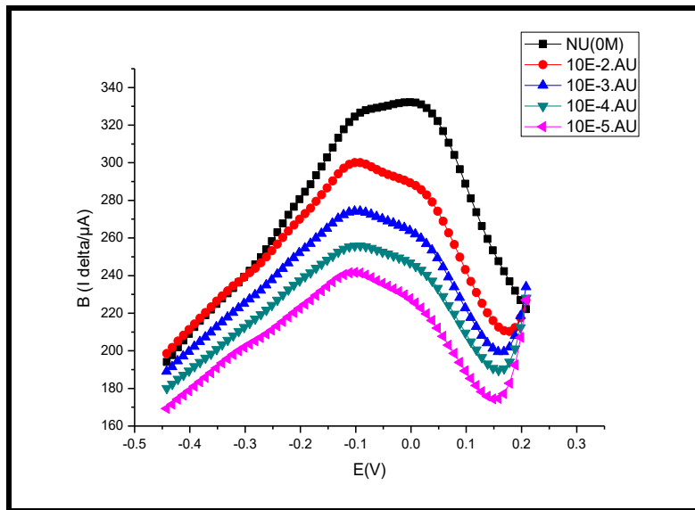
Figure III.14: Voltamogrammes de SQW relatives à la détection de A.URIQUE dans un milieu de PBS (0,1M), pH=7 par la technique MIPs.
